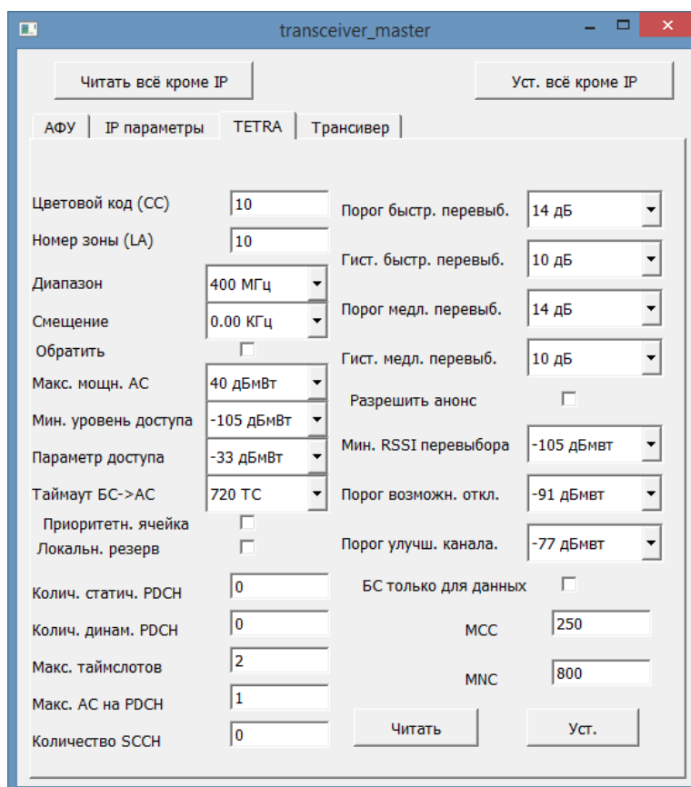
Рисунок 2 Вид главного окна программы
